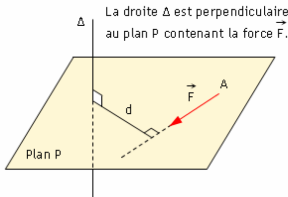
Visualiser l'axe \Delta et la force \vec{F} dans l'espace
